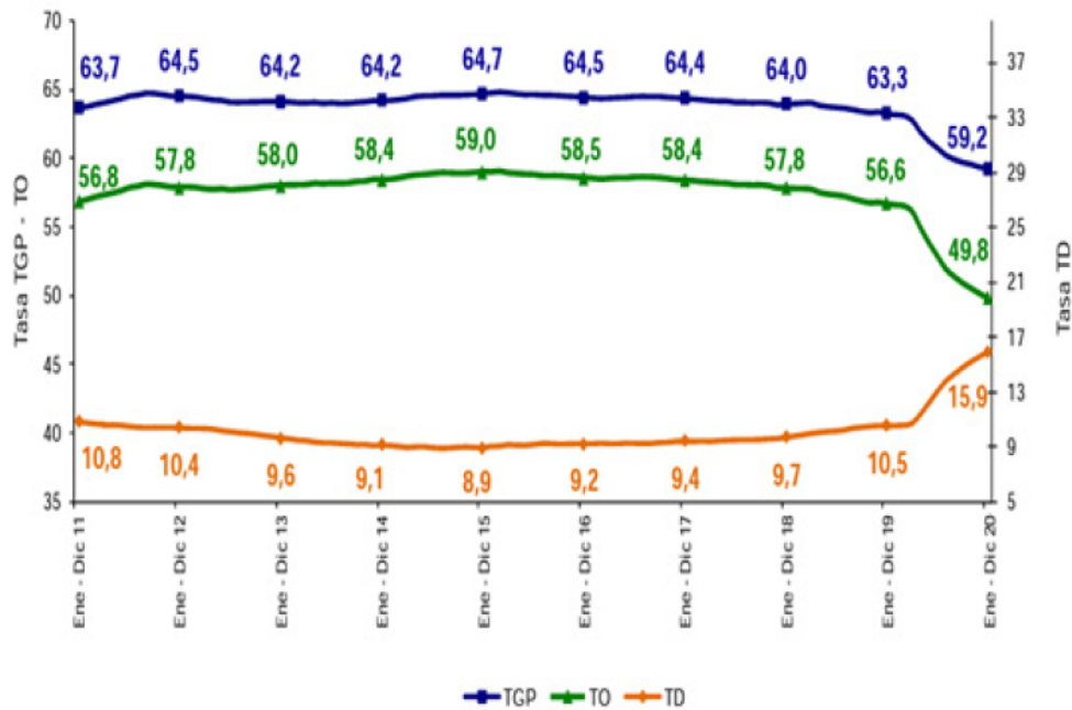
Gráfica 2. Tasa global de participación, ocupación y desempleo total nacional año (2011-2020)
