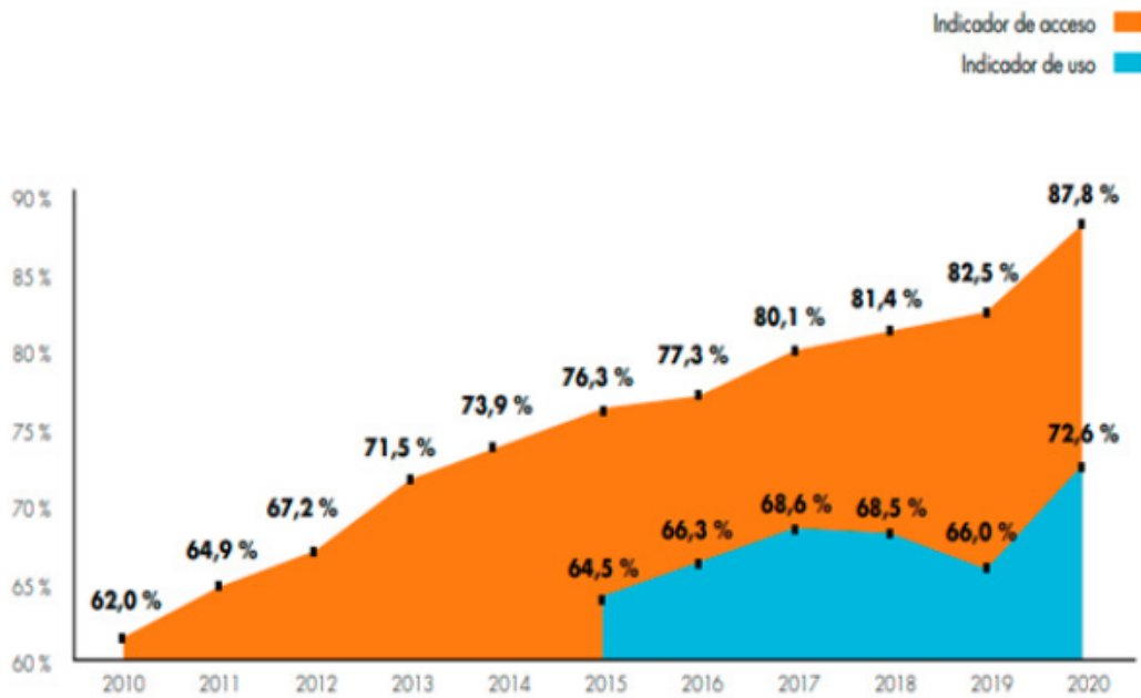
Gráfico 3. Evolución del indicador de acceso 2010-2020
