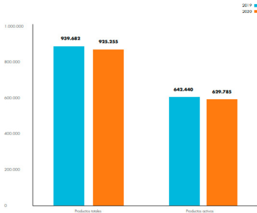
Gráfica 4. Número de personas jurídicas con productos financieros (2019-2020)
