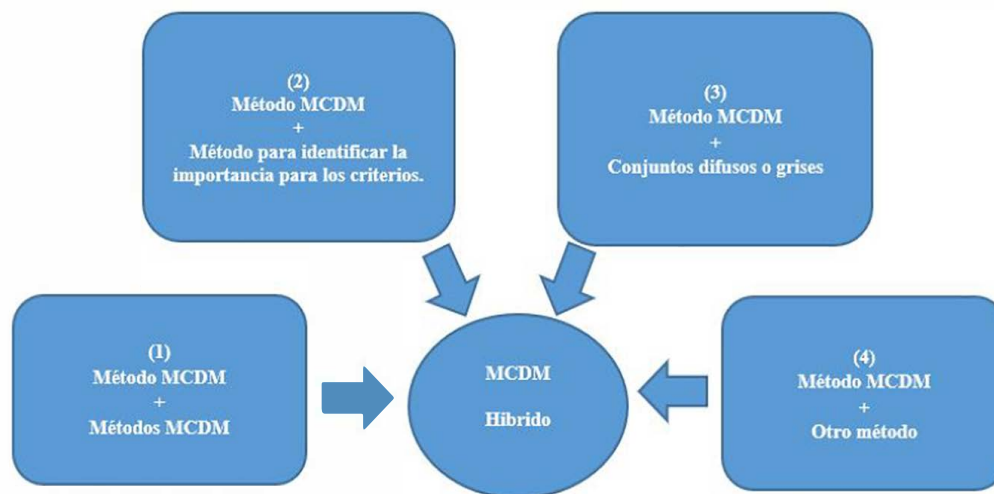
Figura 3. Composición del método híbrido MCDM recurso tomado de peng et al,2016)
