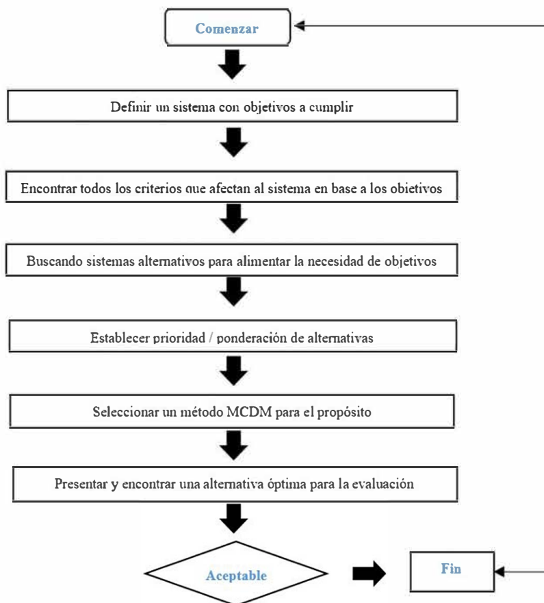
Figura 2. Procedimiento general de la técnica MCDM.(Abhishek,2017)
