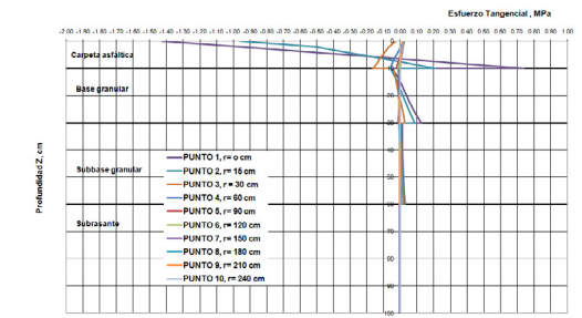
Figura 7. Variación del esfuerzo tangencial de los puntos de estudio
