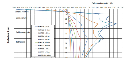
Figura 3. Variación de la deformación radial de los puntos de estudio
