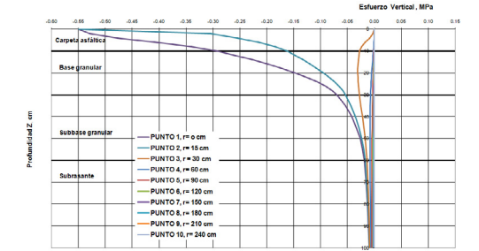
Figura 8. Variación del esfuerzo vertical de los puntos de estudio
