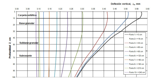
Figura 9. Deflexión de los puntos de estudio
