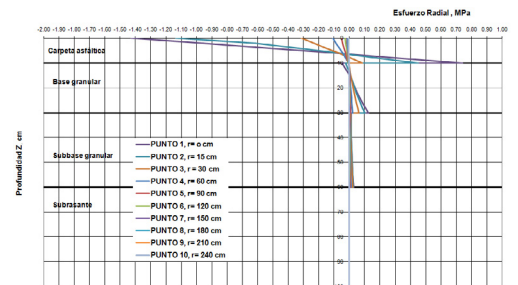
Figura 6. Variación del esfuerzo radial de los puntos de estudio
