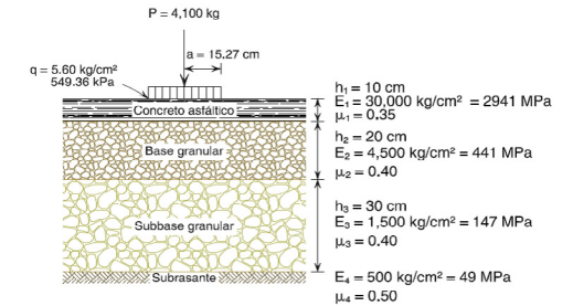
Figura 1. Modelo estructural de referencia de pavimento
