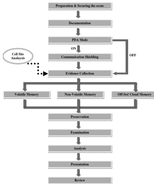
Figura. 5: Modelo de investigación forense para teléfonos inteligentes. Fuente: (Goel, 2012)
