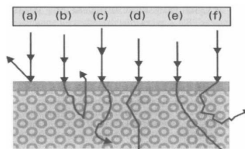
Figura 1. Radiación infrarroja. (a) Reflexión; (b) reflexión difusa; (c) absorción; (d) transmisión; (e) difracción; (f) difusión Fuente: Givens et al., 1997
