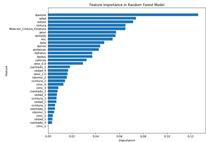
Figura 3. Importancia de características en el modelo Random Forest.
