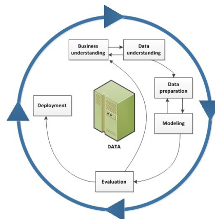
Figura 1. Diagrama CRISP-DM [18]
