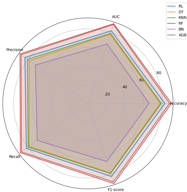
Figura 2. Comparación de Modelos en Predicción de Hipertensión (Gráfico de Radar)
