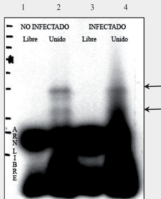
Figura 2. Ensayos de entrecruzamiento UV de ARN 5' UTR-Proteínas de maíz. ARN marcado incubado en ausencia (líneas 1 y 3) o presencia (líneas 2 y 4) de extractos proteicos de maíz. Las flechas al costado derecho indican los complejos ARN – proteína.
