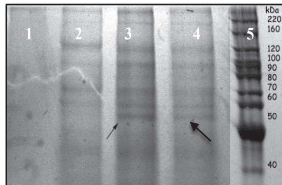
Figura 4. Gel SDS-PAGE con proteínas eluidas. En el carril 1 control sin ARN, carril 2 control con ARNt, carriles 3 y 4 eluidos 1 y 2, carril 5 marcador de peso molecular. En los carriles 3 y 4 se visualiza una banda de aproximadamente 53 kDa que no está presente en el carril 2, en el que se empleó ARNt como control positivo, ni en el carril 1, control en el que no se cargó ARN. En el carril 5 marcador de peso molecular. Fuente: Autor
