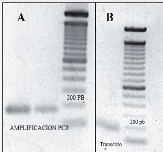
Figura 1. A. RT-PCR de la región 5' UTR de SCMV. B. Transcrito de la región 5' UTR. Tanto los productos de RT-PCR como el transcrito presentan el tamaño esperado
