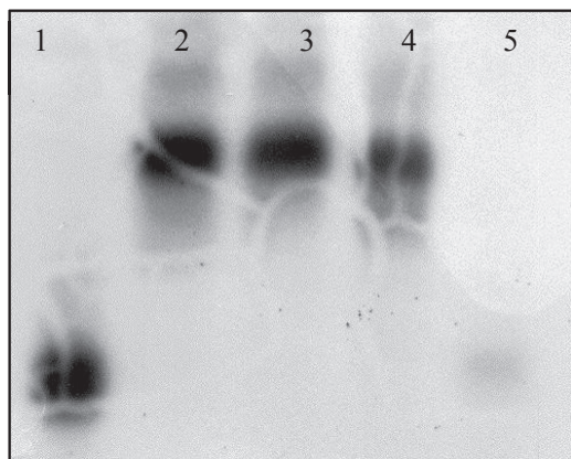
Figura 3. Estabilidad de los complejos 5' UTR. Los Complejos ARN-proteína formados por UV fueron tratados con KCl 0.3 M (Línea 3) 0.6M (Línea 4) y proteínasa K (Línea 5). En la línea 1 ARN marcado libre. Línea 2 ARN unido a proteína sin tratamiento de sal Foto: Autor
