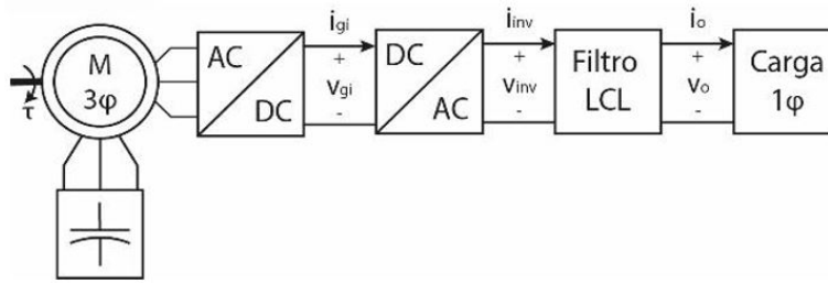
Figura 2. Esquema VRFT modificado
